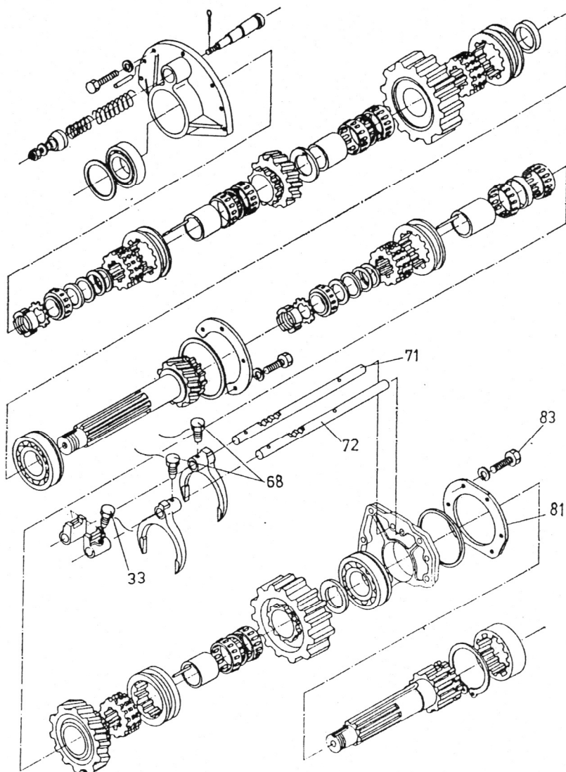
77.ábra: Hajtóműház szerelvényei
